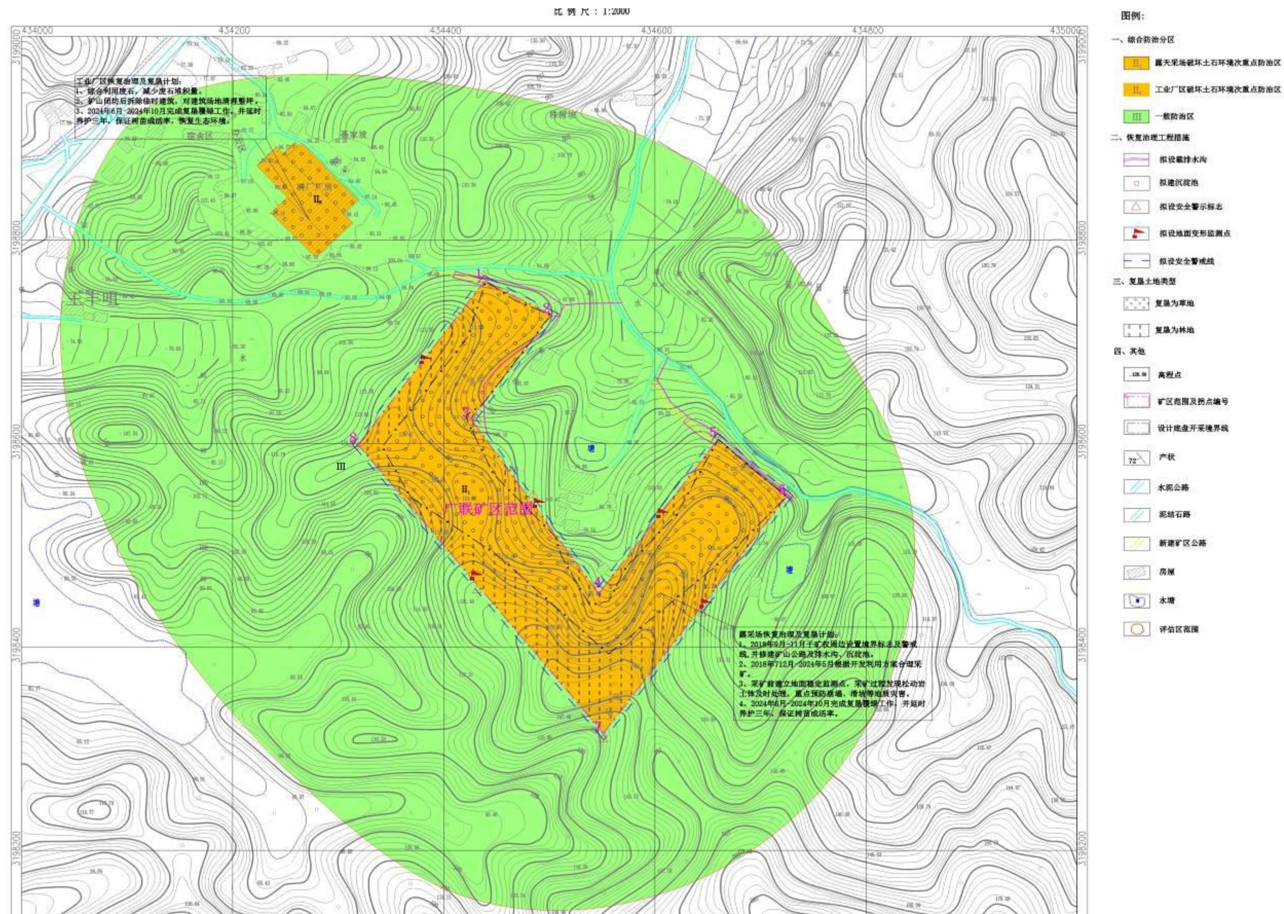
附图3 项目矿山地质环境综合防治工程部署图
