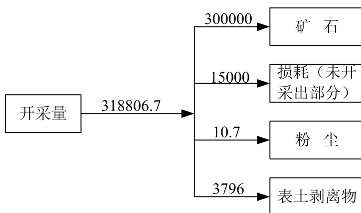
图 5-2 项目矿山开采过程物料平衡（t/a）
