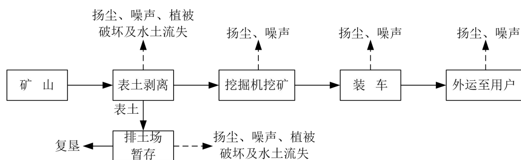
图 5-1 营运期生产工艺流程及产污环节图
