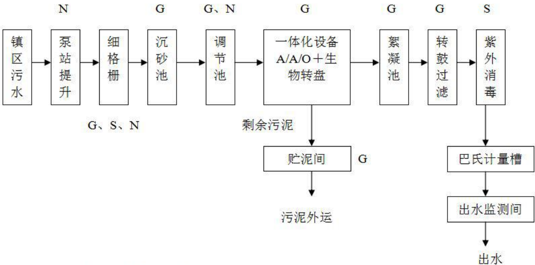
图4 污水处理工艺流程及产污节点图
