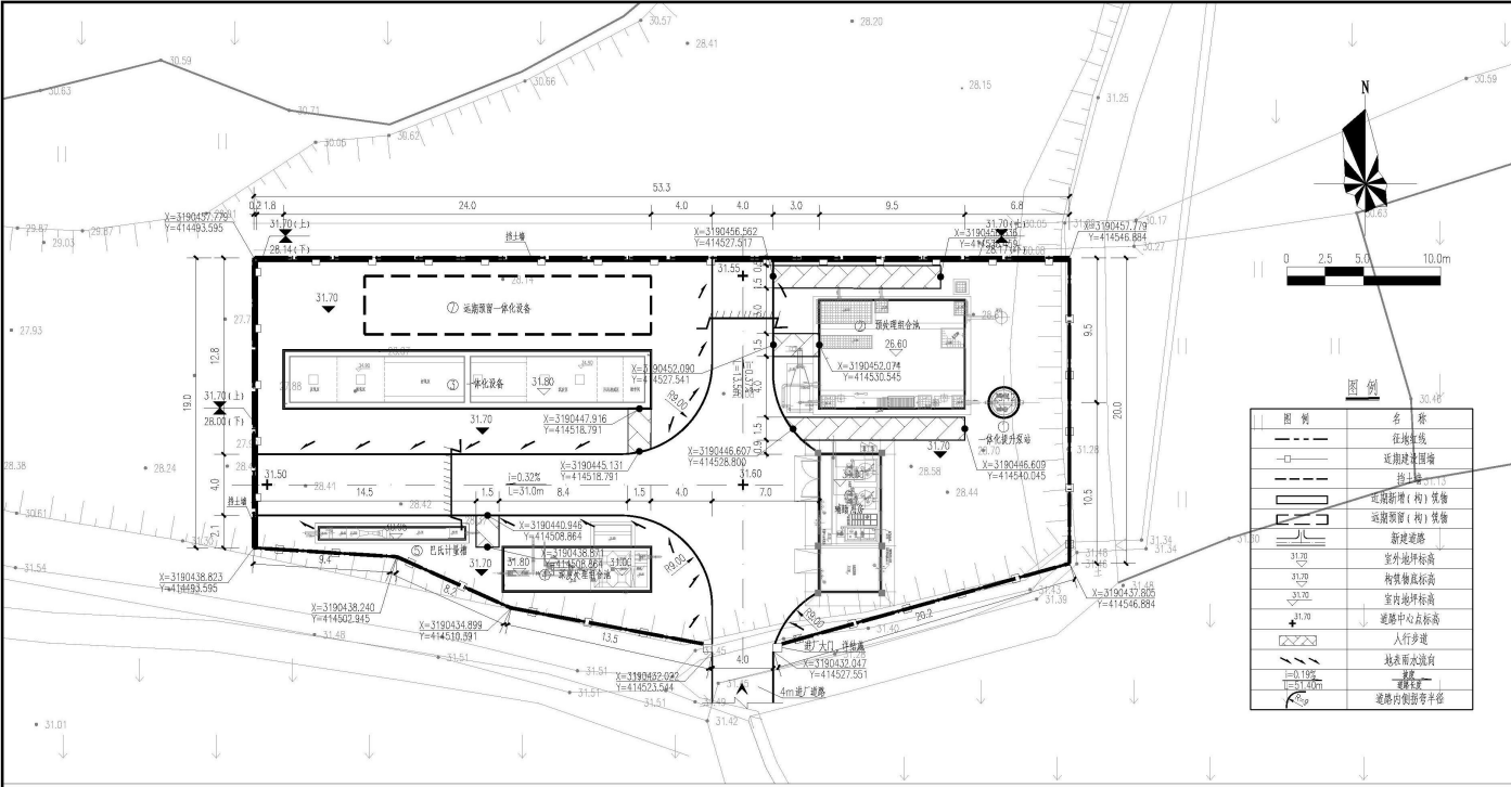
芙蓉集镇污水处理厂竖向布置图 1:200
