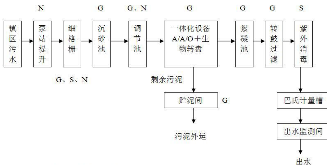
图4 污水处理工艺流程及产污节点图
