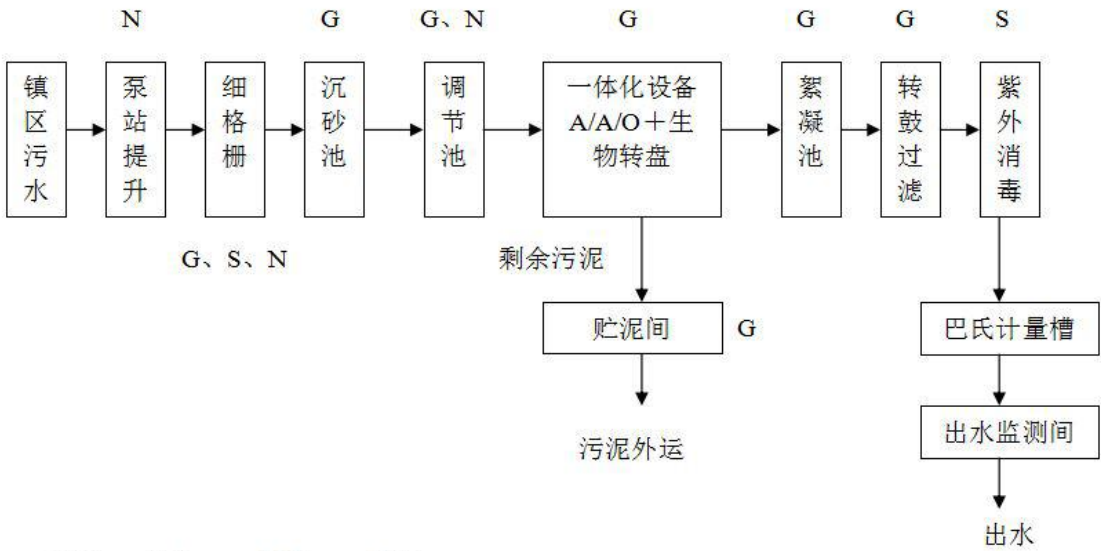
图 4 污水处理工艺流程及产污节点图
