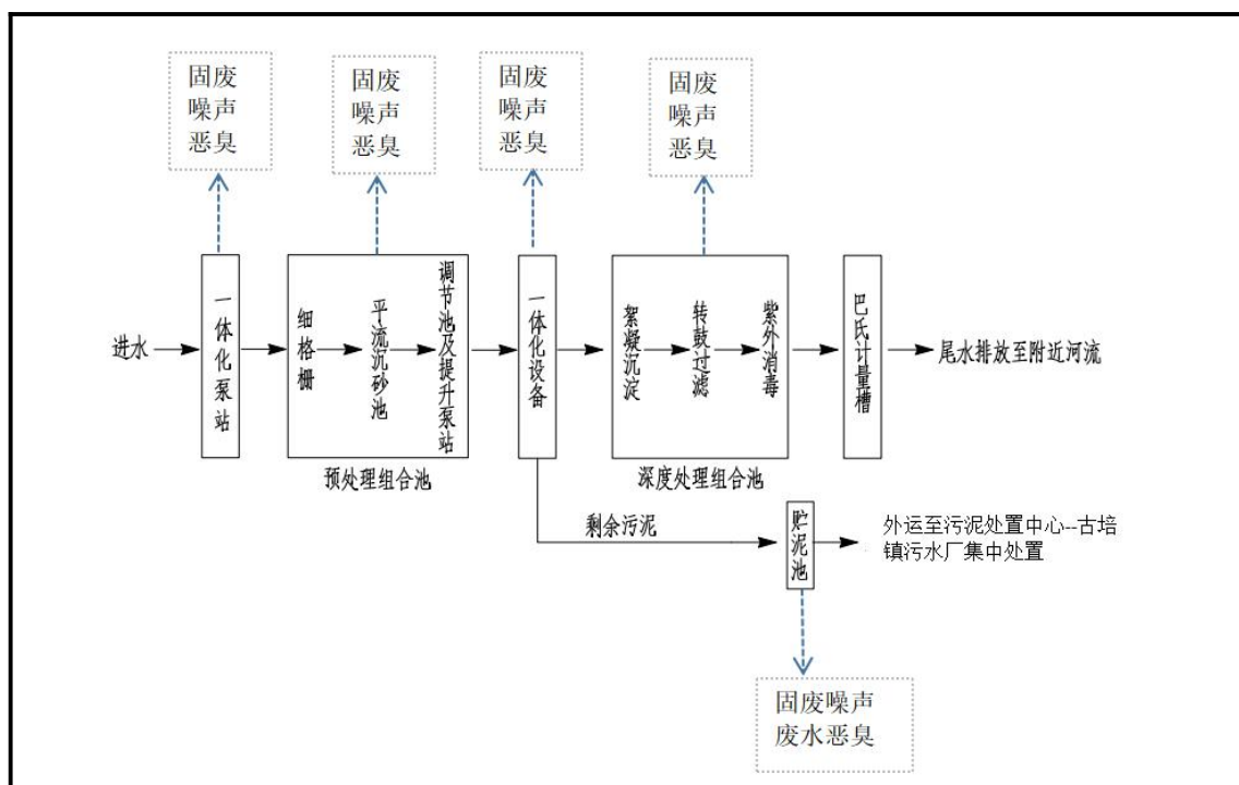
图 1-1 本项目污水处理工艺流程示意图
