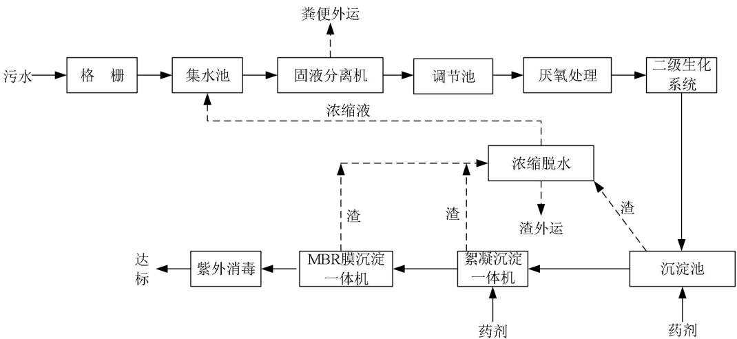
图 7.2-1 污水处理工艺流程图
