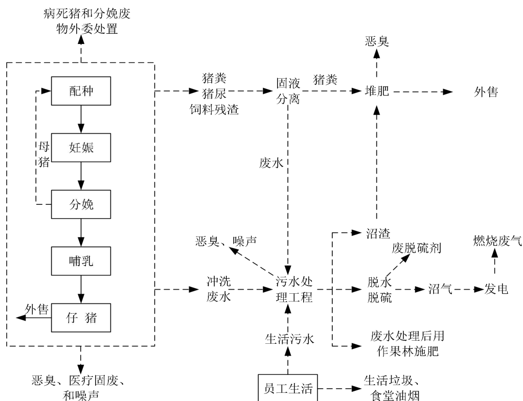
图 3.4-1 养殖工艺流程及排污节点图
