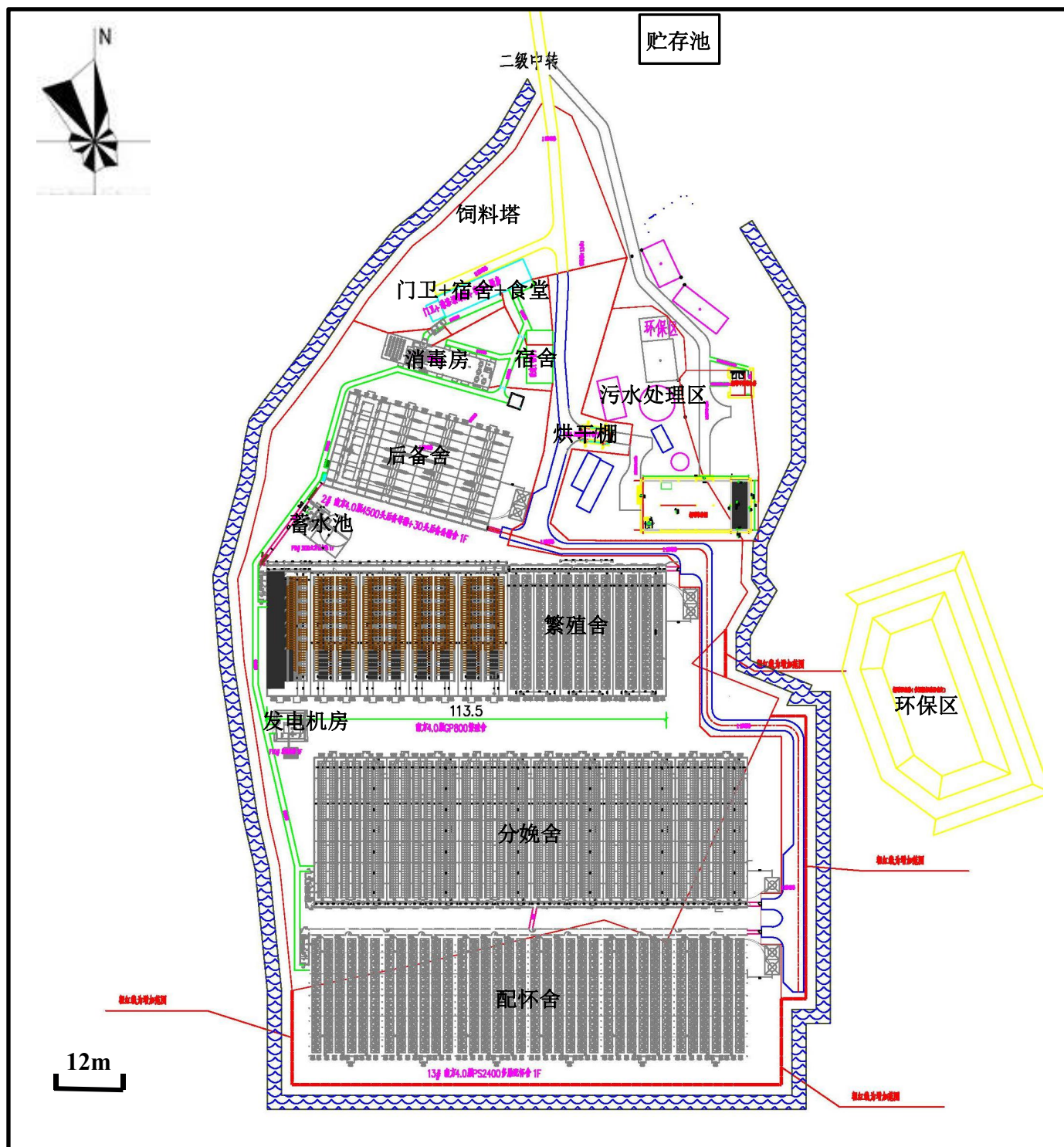
附图2 一期养殖区及污水处理区平面布局图
