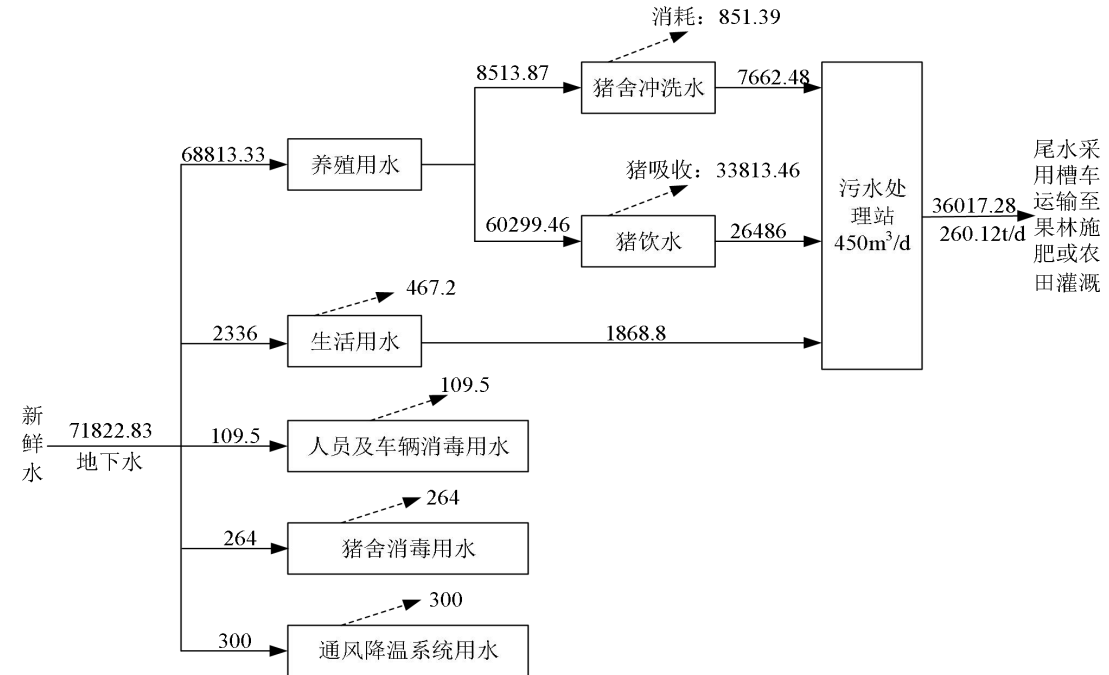
图 4.5-1 工程水平衡图 单位：m³/a
