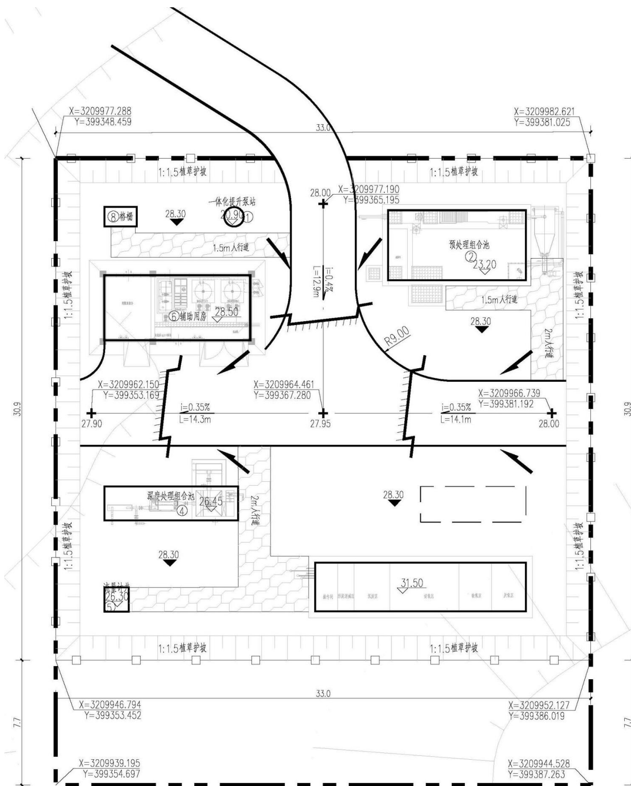
附图 2 项目厂区平面布置图
