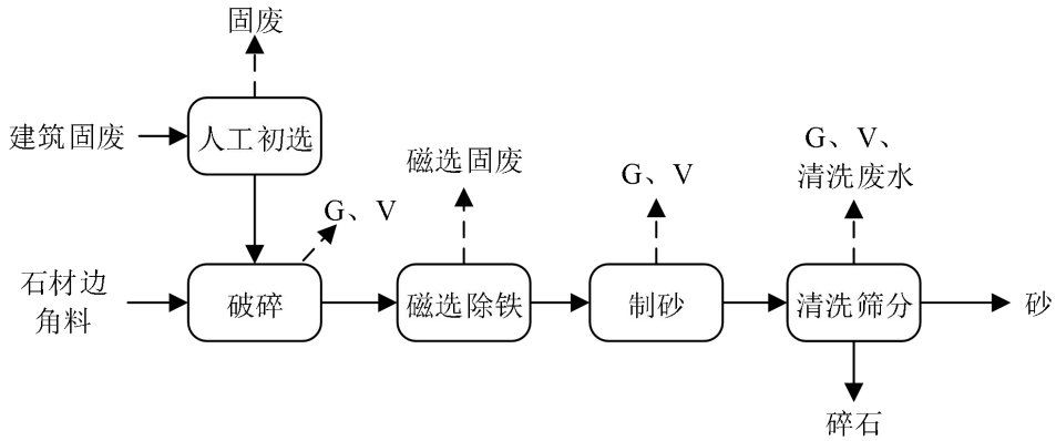
图 2-4 工艺流程图
