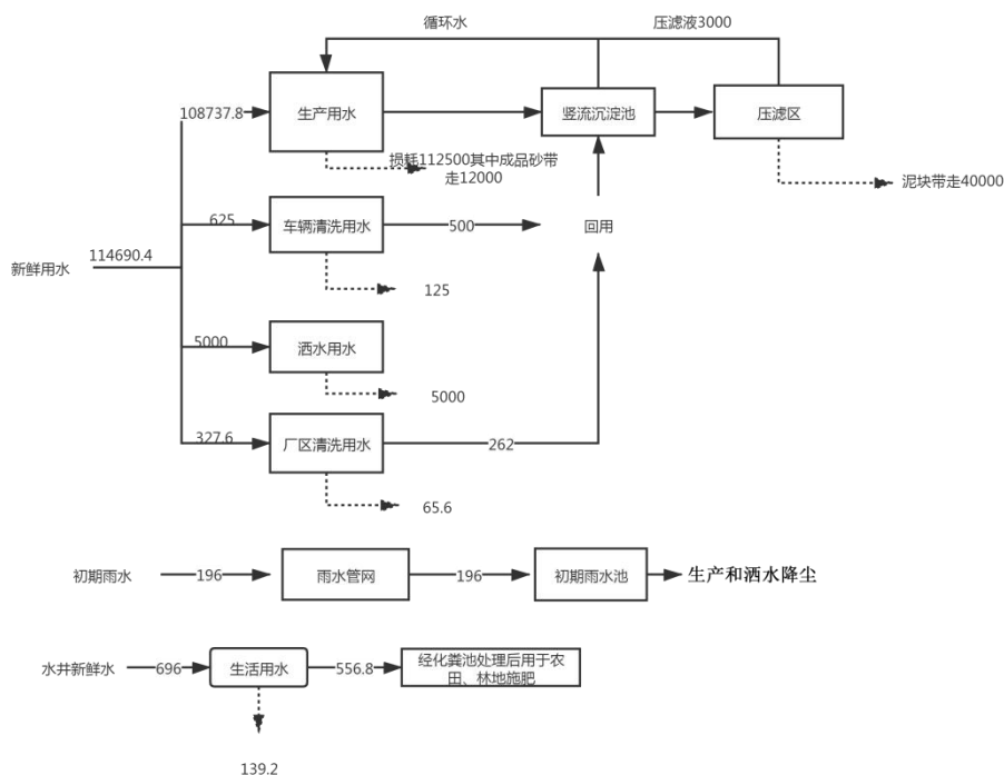
图 2-2 水平衡图（最大用水量，单位：m 3 /a, 初期雨水 m 3 /次）
