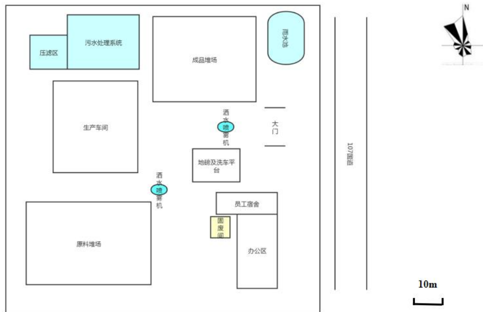
图 2-1 平面布置图
