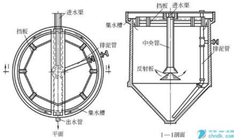
图 4-1 竖流沉淀池示意图
