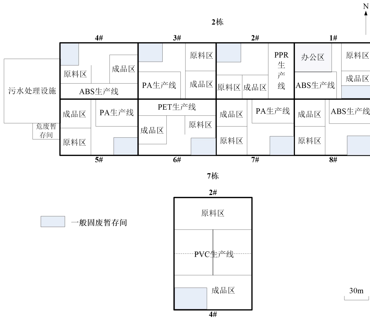
附图三 平面布局图
