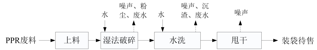
图 2-4 2 栋 2#车间 PPR 生产工艺流程图
