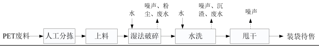
图 2-8 2 栋 8#车间 ABS 工艺流程图
