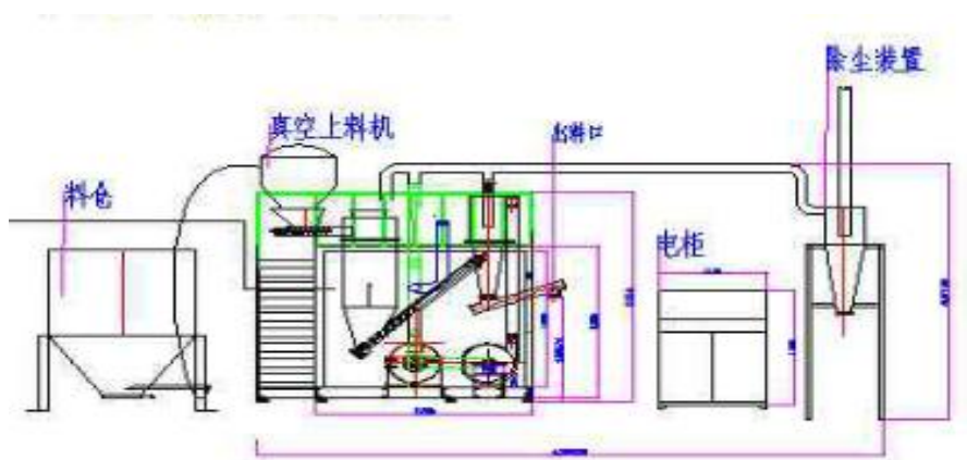
图 4-1 磨粉机示意图
