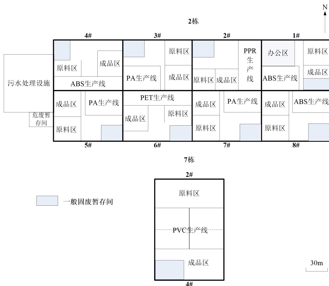
图 2-1 平面布局图
