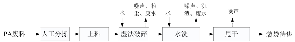
图 2-5 2 栋 3#、5#、7#车间 PA 工艺流程图
