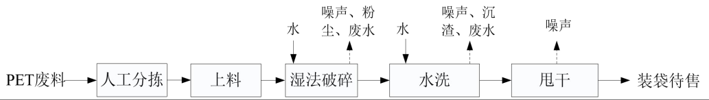
图 2-7 2 栋 6#车间 PET 工艺流程图
