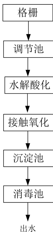
图 4-1 污水处理设施工艺流程图
