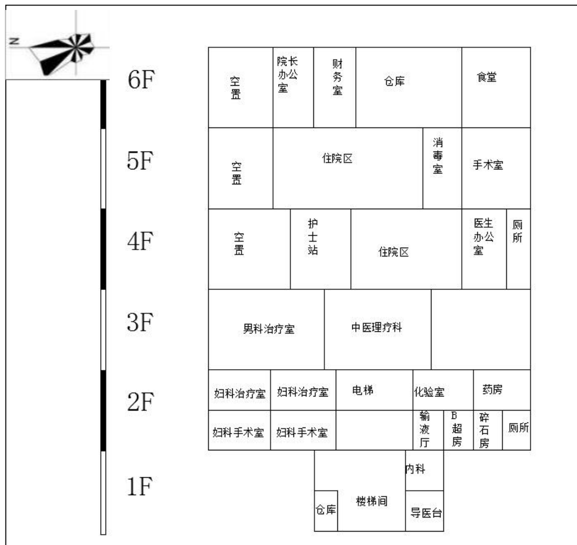
附图 4 1~6 层平面布置图
