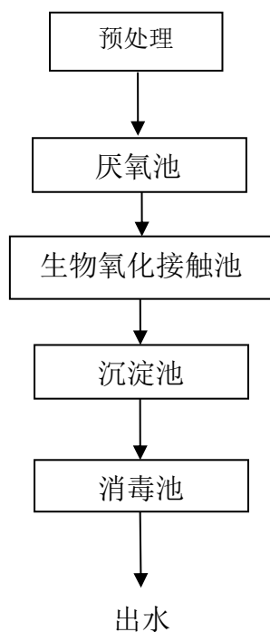
图 4-1 污水处理设施工艺流程图
