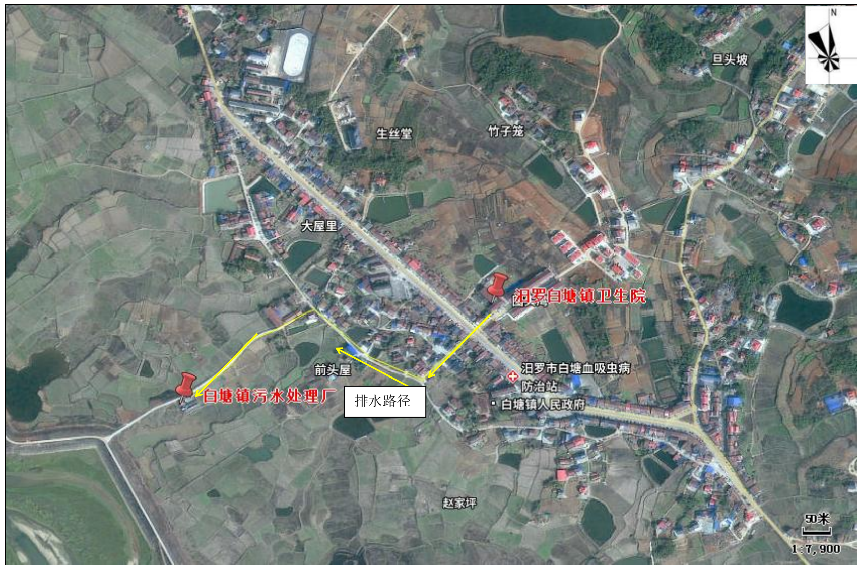
附图 6 项目排水路径图
