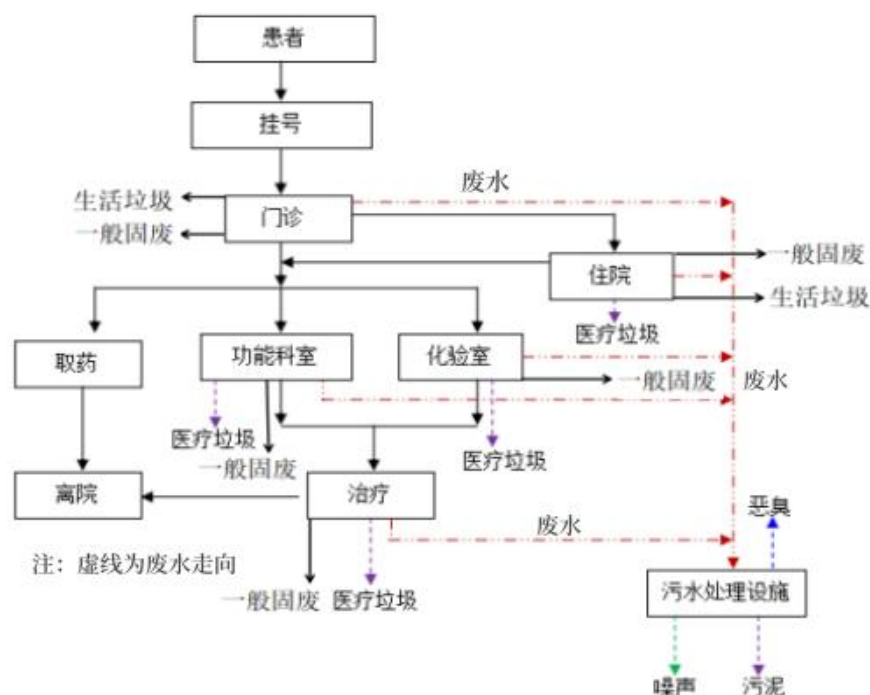
图 2-1 项目营运期工艺流程及产污环节示意图
