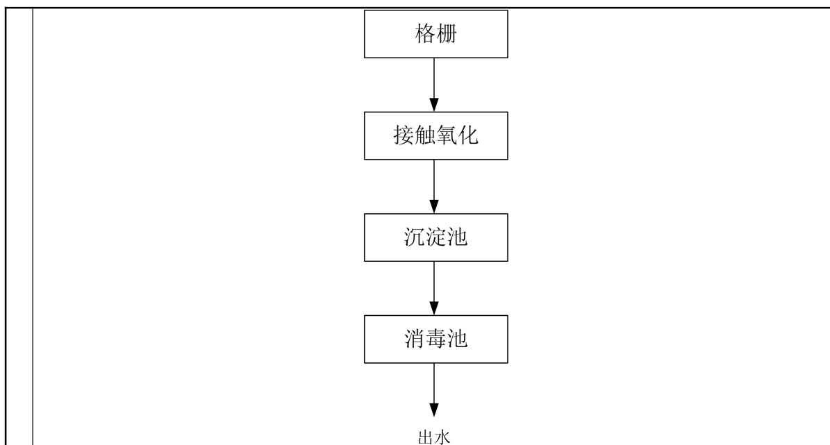
图 4-1 污水处理设施工艺流程图
