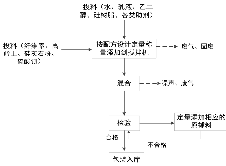
图 2-5 防水涂料生产工艺流程图
