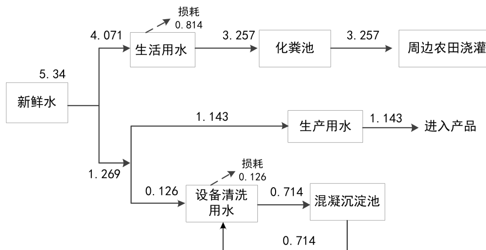
图 2-1 水平衡图 (单位: m 3 /d)
