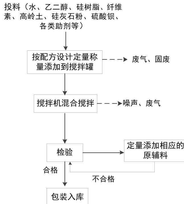
图 2-4 仿石漆涂料生产工艺流程图
